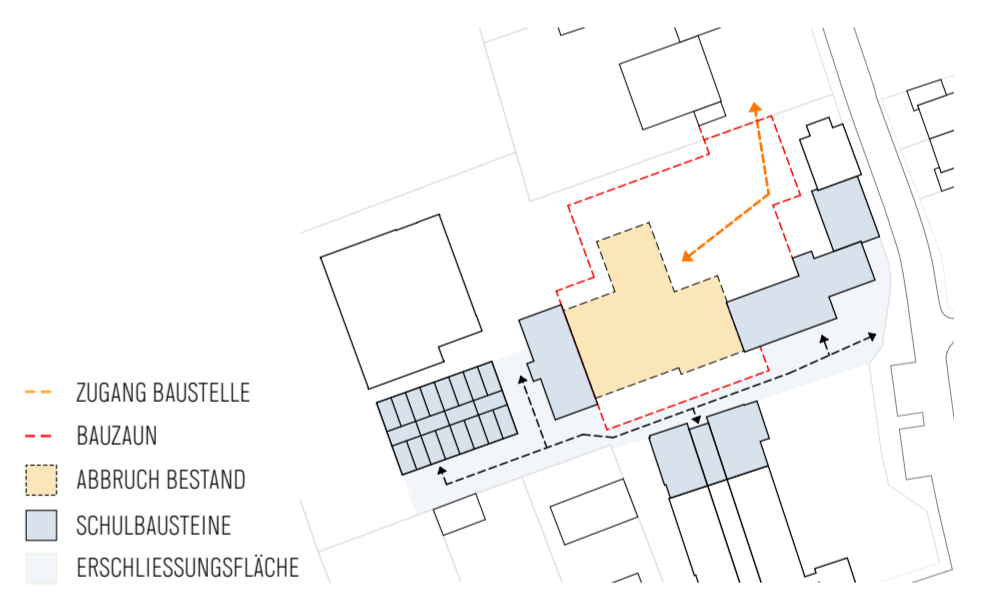
BAUSTUFE 2 - ABBRUCH BESTAND
