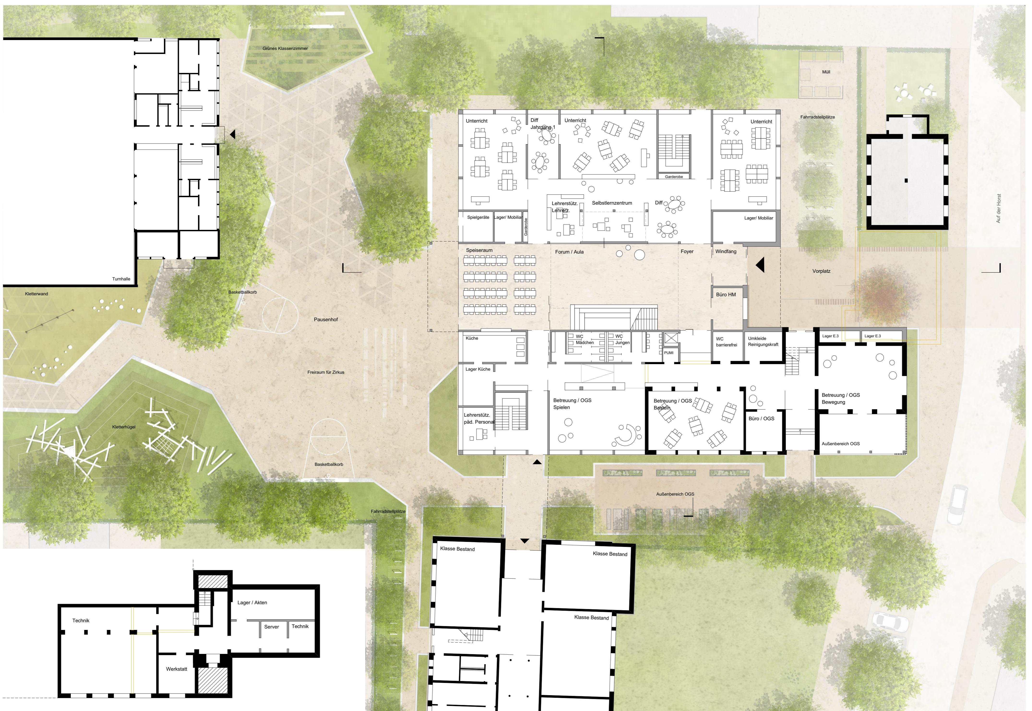
Grundriss UG 1:200
