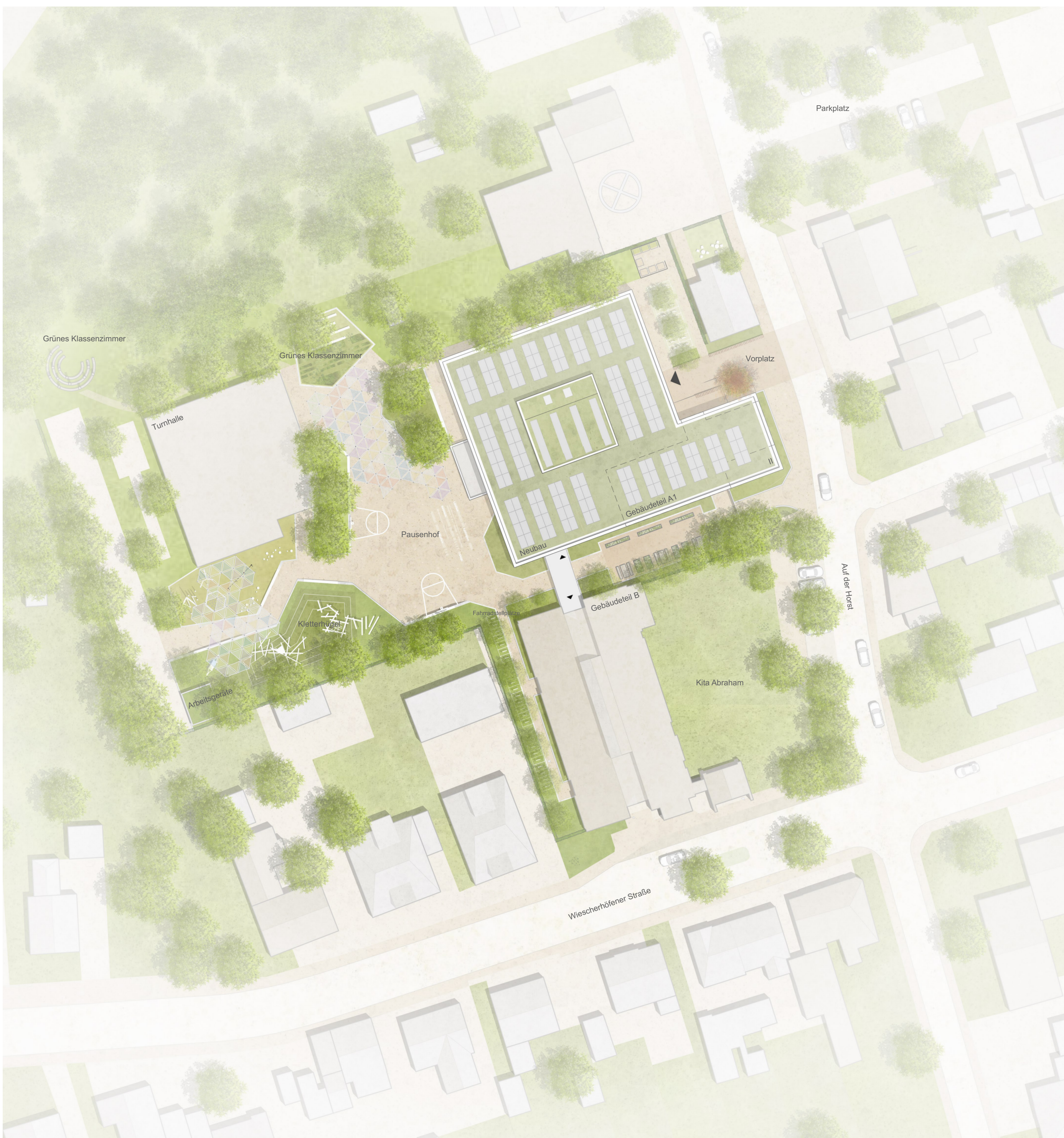
Lageplan 1:500
